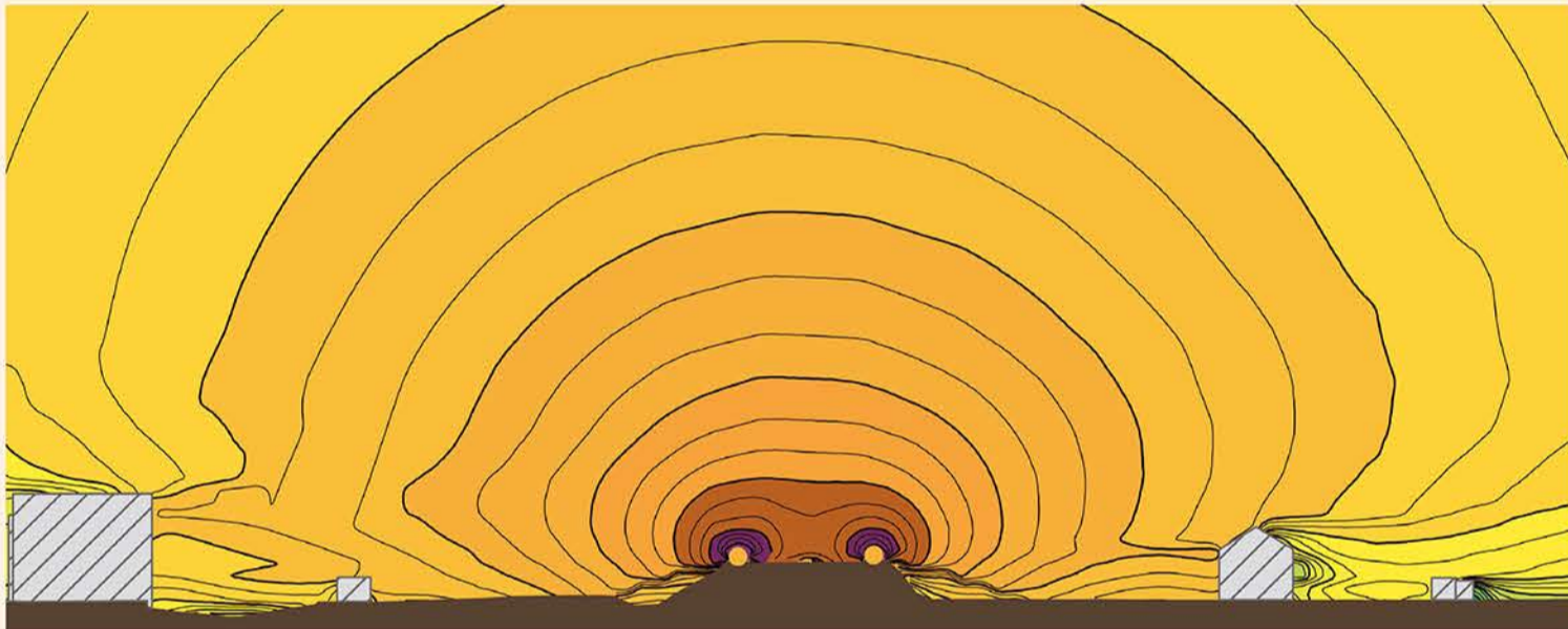
Damm
